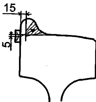
Рисунок 4 - Схемы прозвучивания и зоны контроля цельнокатанных колес при варианте метода DR3.3
