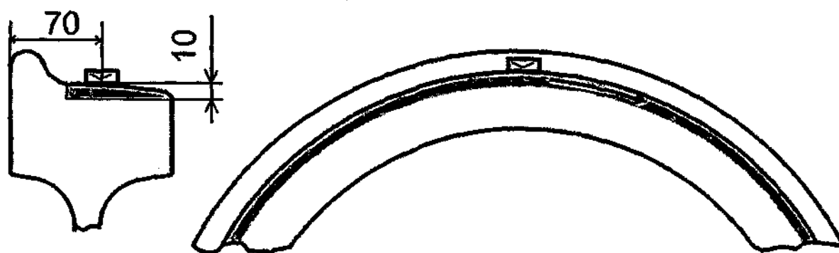
Рисунок 5 - Схема прозвучивания и зона контроля цельнокатанных колес при варианте метода DR4
