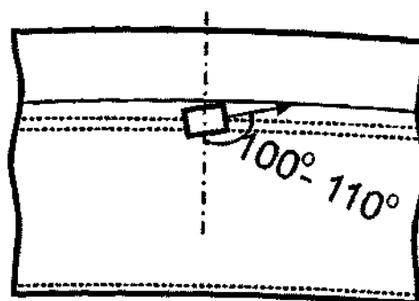
Рисунок 4 - Схемы прозвучивания и зоны контроля цельнокатанных колес при варианте метода DR3.3
