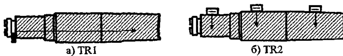
Рисунок 12 – Схемы прозвучивания осей колесных пар при вариантах методов TR1 и TR2
