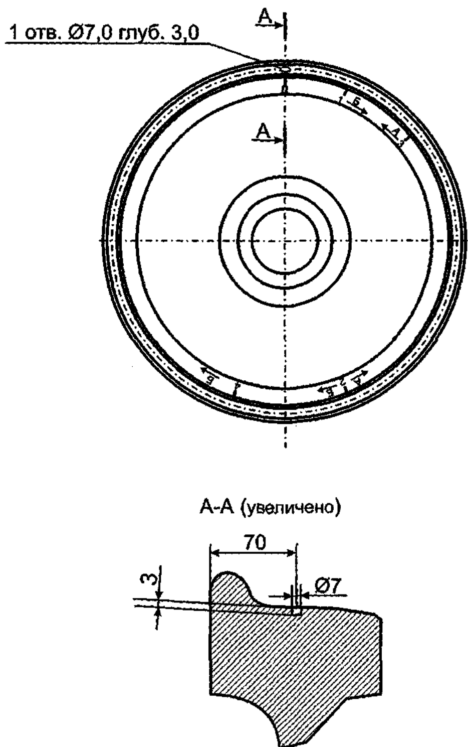
Рисунок ПА.6 – Эскиз рекомендуемого настроечного образца для УЗК цельнокатаных колес по варианту метода DR4
